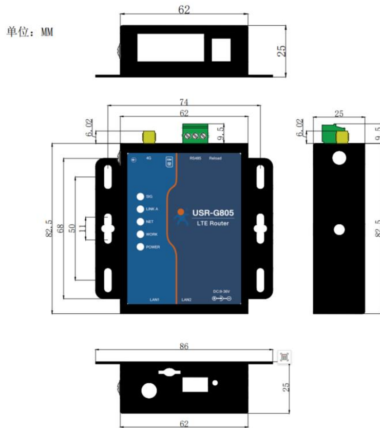
USR-G805 产品尺寸
