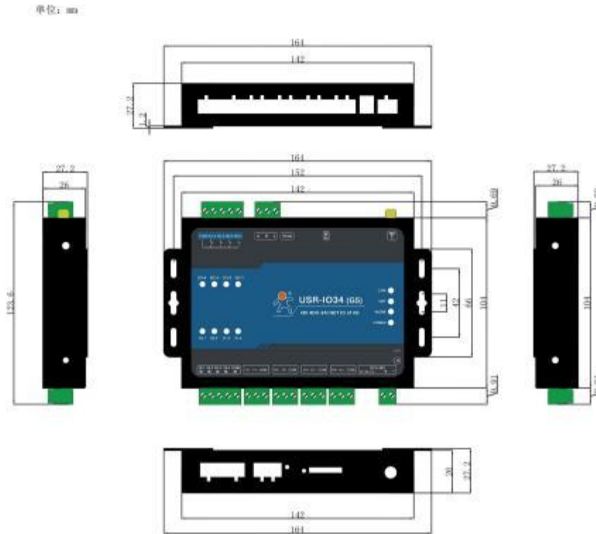
图 15 USR-IO34-G5 尺寸图
